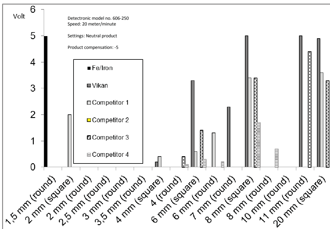
1c. Podsumowanie przeprowadzonych badań w celu sprawdzenia wielkości fragmentów wykrywalnych przez detektory metali, dostarczanych w przemyśle spożywczym. (Vikan/Detectronic, 2012).
